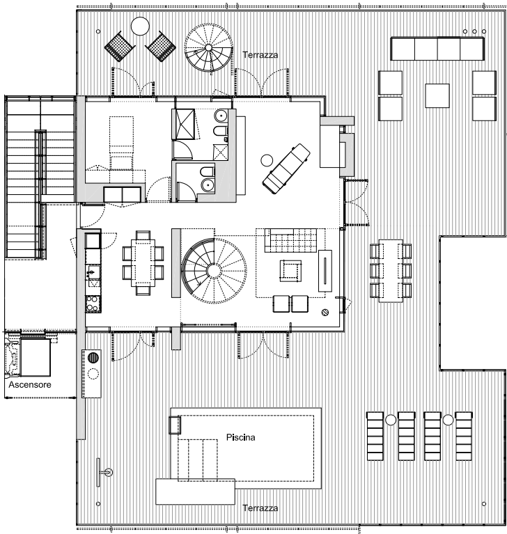
Piano Inferiore
